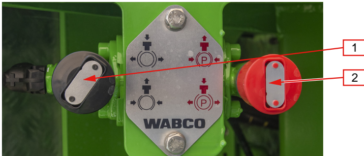
Abb. 40. Doppellöseventil
