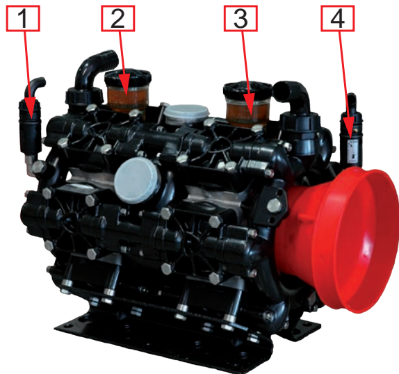
Abb. 34. Flüssigkeitspumpe AR 500
