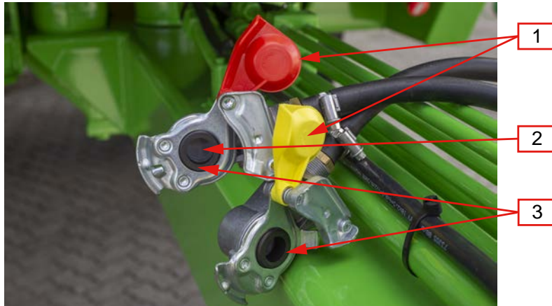
Abb. 42. Pneumatikkupplungen
