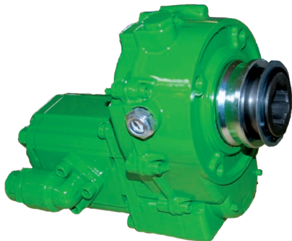
Abb. 35. Aufsteckpumpe Profi-Class
