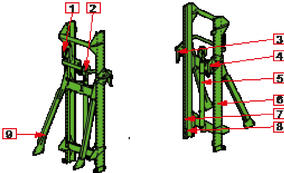
Abb. 10. Hubmast
