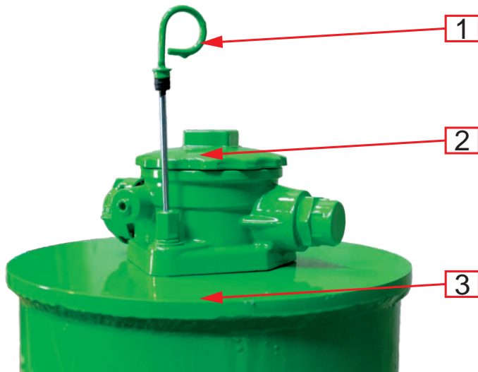
Abb. 36. Hydrauliktank Profi-Class mit Aufsteckpumpe
