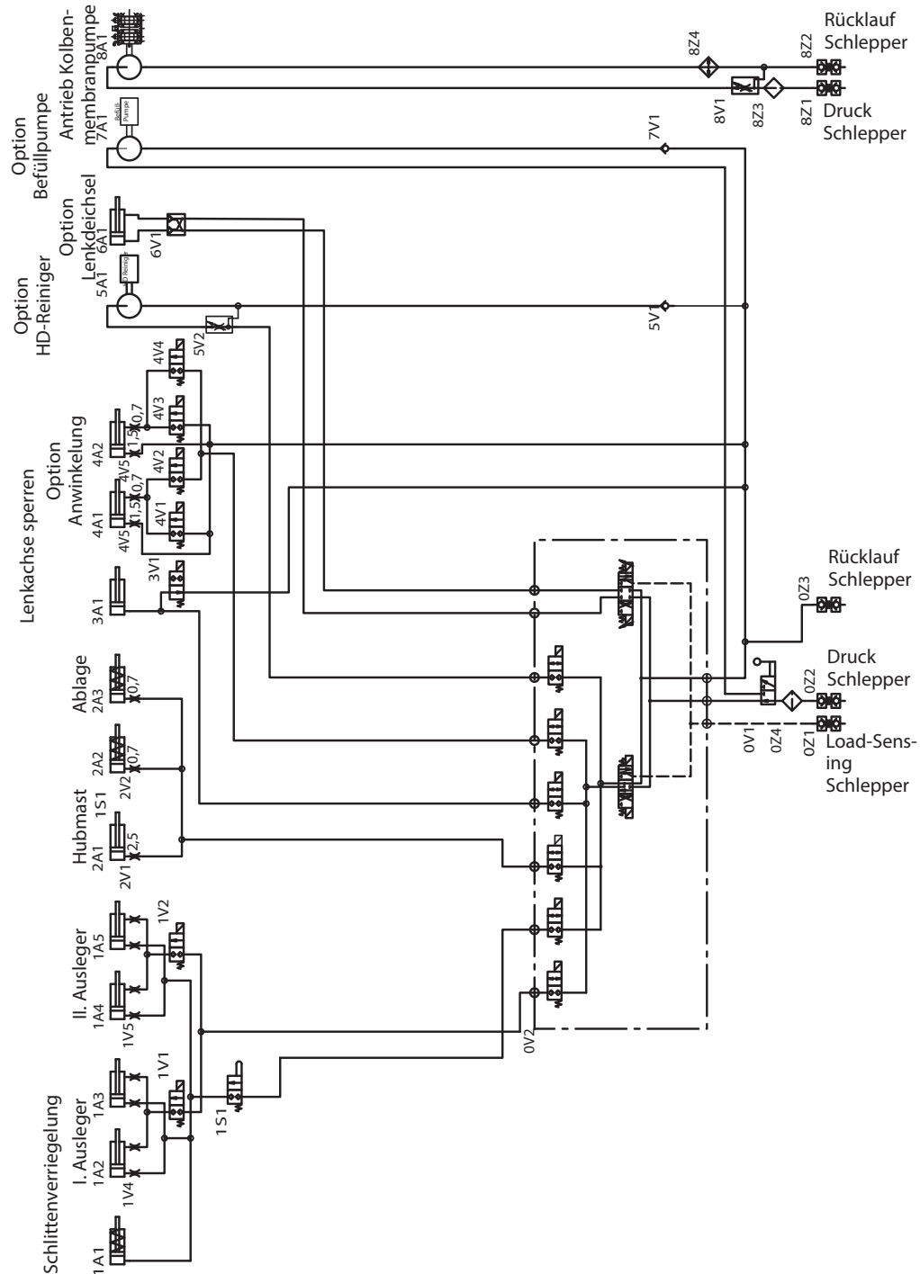
Abb. 132. Hydraulikplan mit Steuerblock Pumpenantrieb über Zugmaschine Profi-Class
