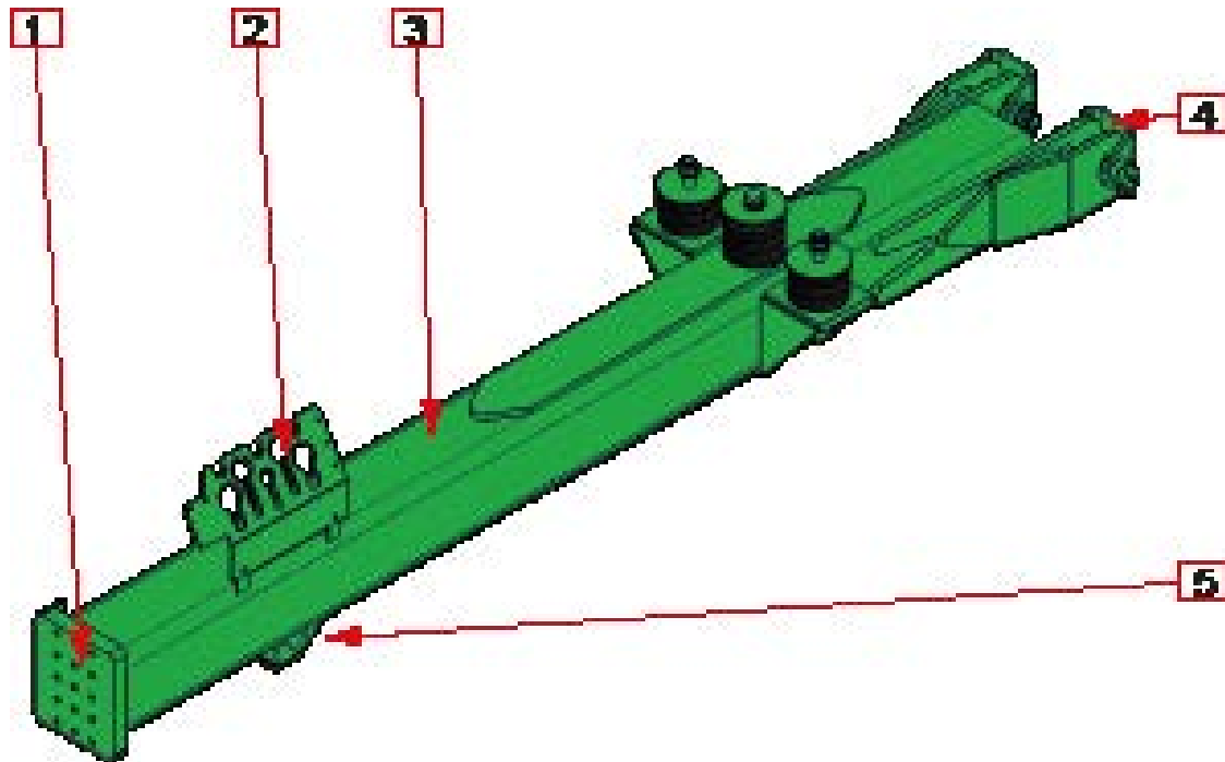
Abb. 6. Starre Deichsel
