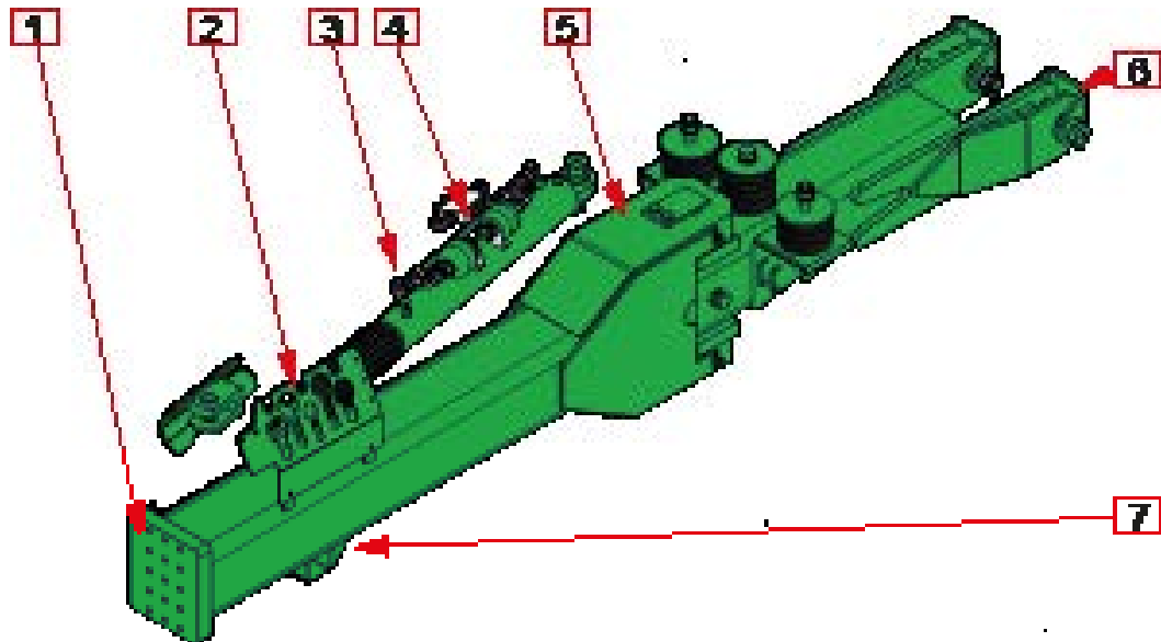
Abb. 7. Lenkdeichsel
