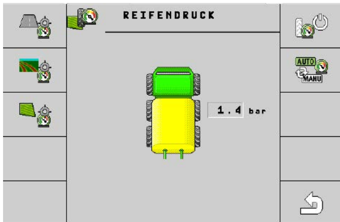
Abb. 73. Manueller Modus
