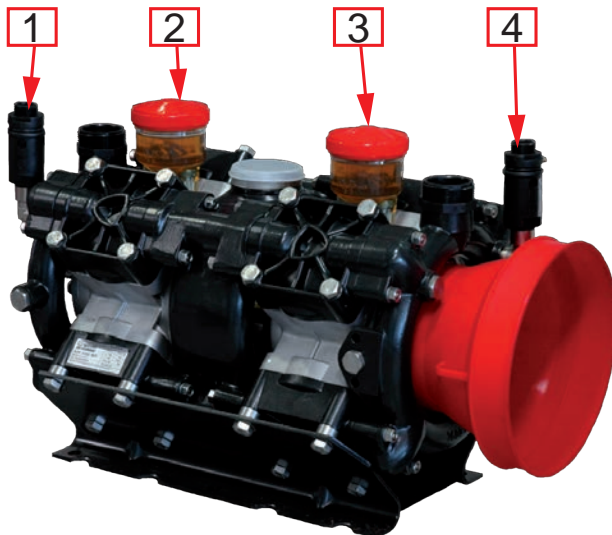
Abb. 33. Flüssigkeitspumpe AR 320
