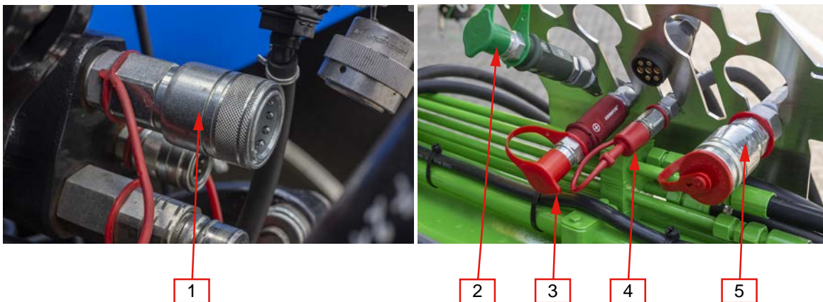
Abb. 41. Hydraulikkupplungen
