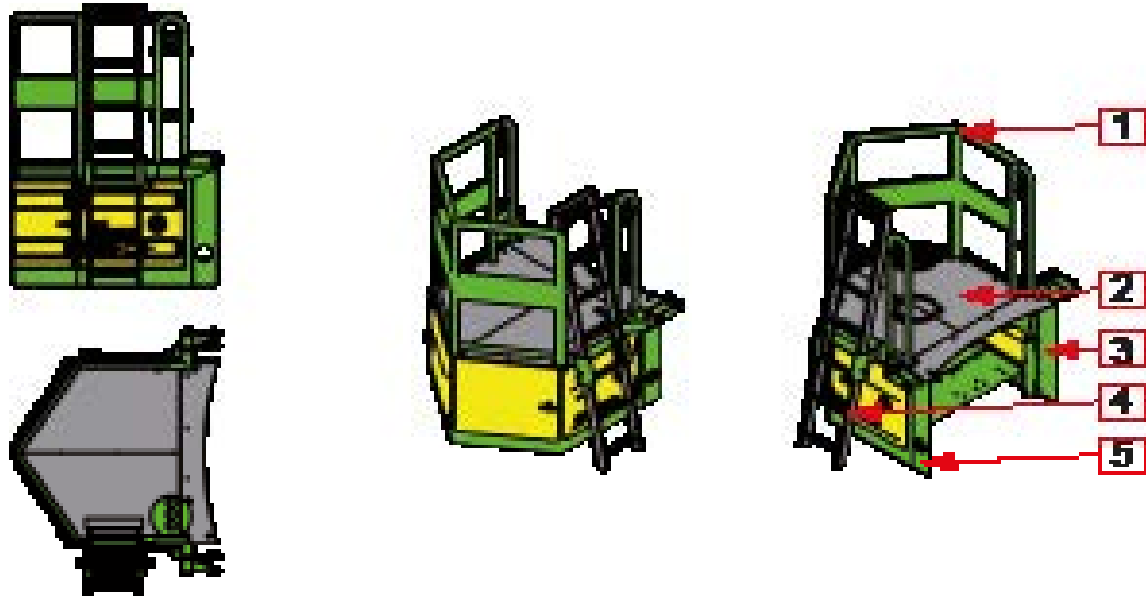
Abb. 4. Vorbau Profi-Class
