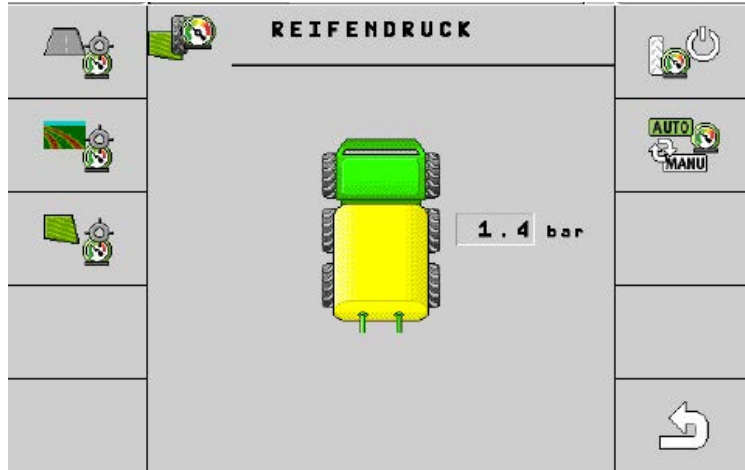
Abb. 69. Funktion der Reifendruckregelanlage
