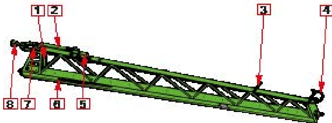
Abb. 15. I. Ausleger
