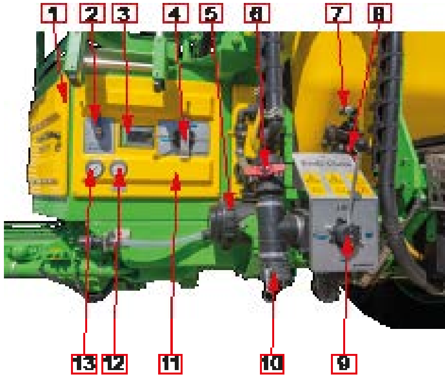
Abb. 27. Übersicht Armaturen und Hähne
