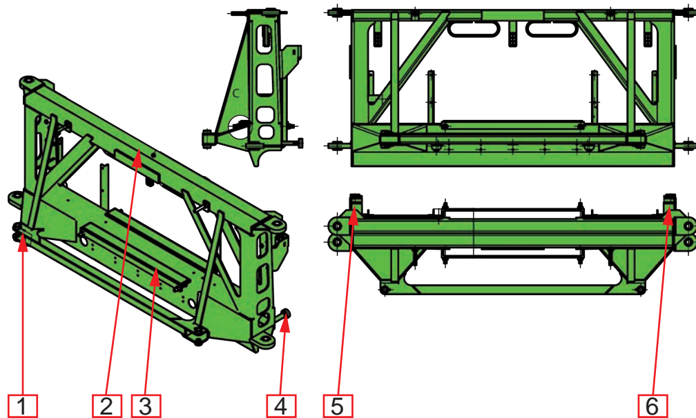
Abb. 14. Mittelrahmen
