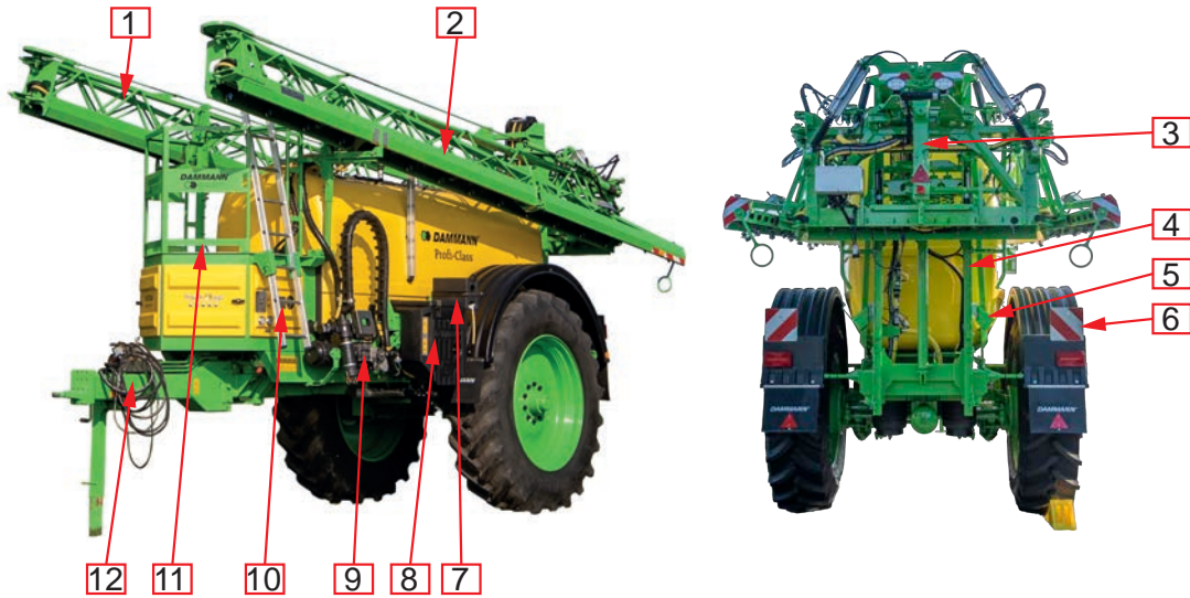
Abb. 3. Geräteübersicht
