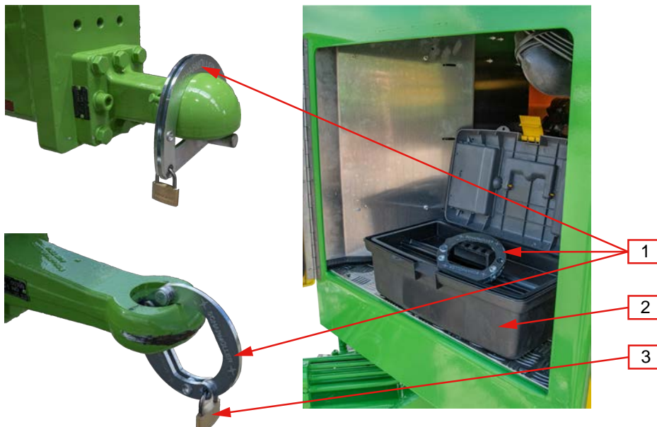
Abb. 55. Sicherung gegen unbefugte Nutzung
