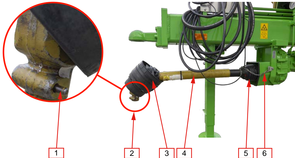
Abb. 54. Gelenkwelle montieren (Beispiel an einer Aufsteckpumpe)
