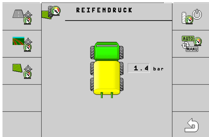
Abb. 70. Maske der Reifendruckregelanlage
