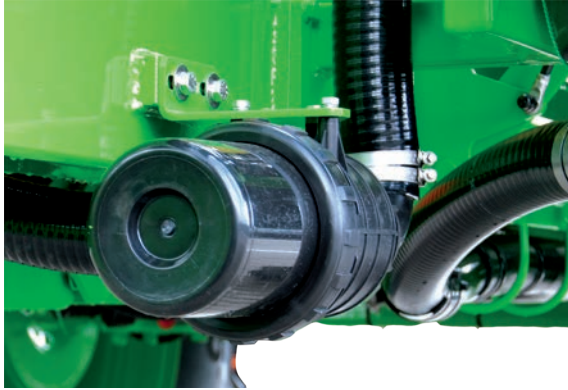
Abb. 105. Saugfilter und Saugfilterschlüssel (rechts)
