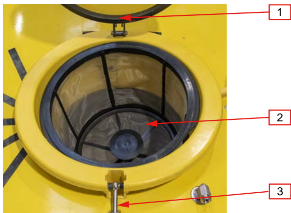
Abb. 60. Befüllung über Einfülldom
