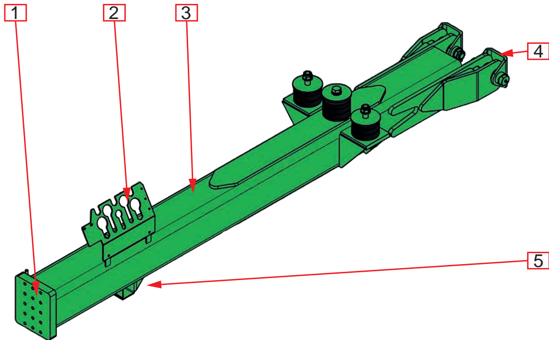
Abb. 6. Starre Deichsel
