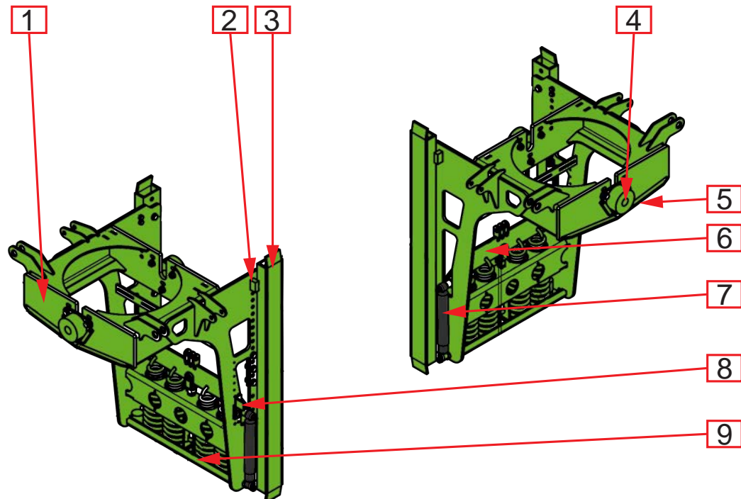
Abb. 11. Schlitten
