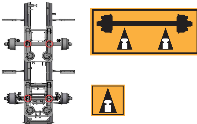
Abb. 129. Wagenheber ansetzen
