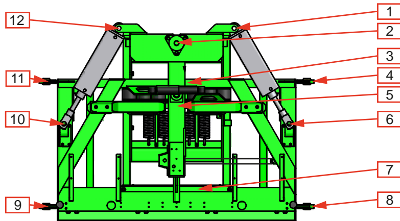
Abb. 121. Schmierplanübersicht Mittelrahmen
