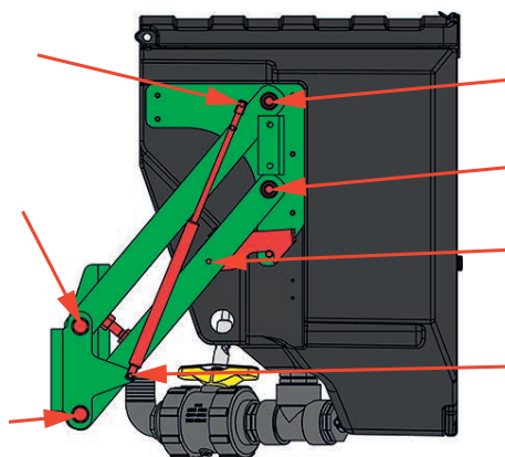
Abb. 119. Schmierplanübersicht Hubmast
