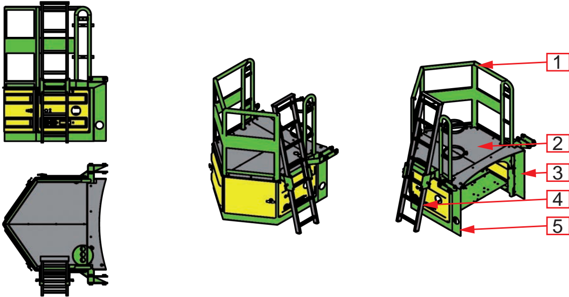
Abb. 4. Vorbau Profi-Class
