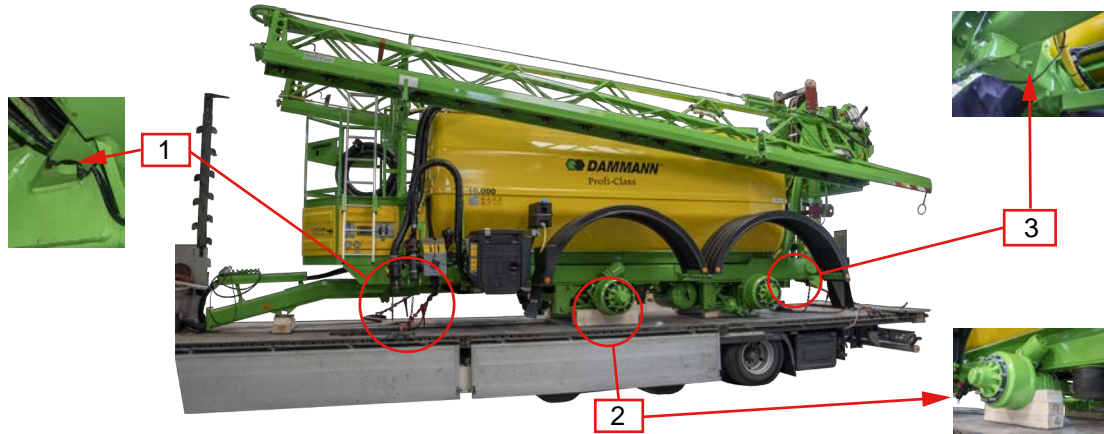
Abb. 52. Verzurren auf einem Tieflader mit Kupplung (Beispiel ANPT)
