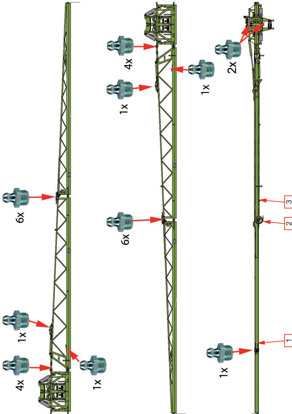
Abb. 124. Schmierplanübersicht Gestänge
