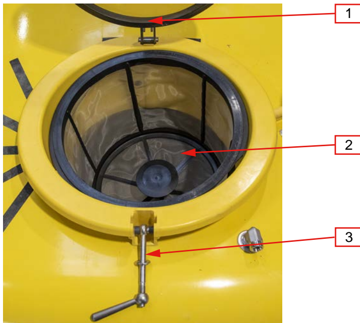
Abb. 61. Einbringen über den Einfülldom
