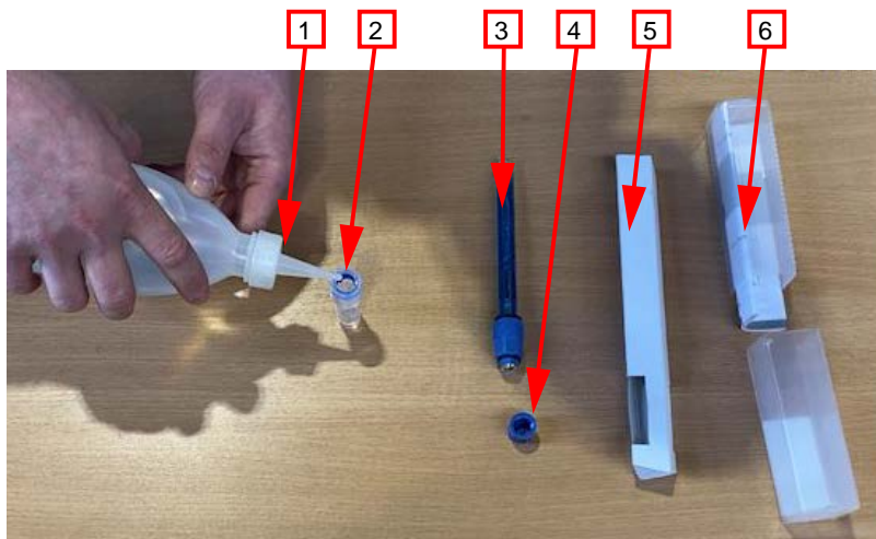
Abb. 103. Zur Aufbewahrung Lösung in Behälter füllen
