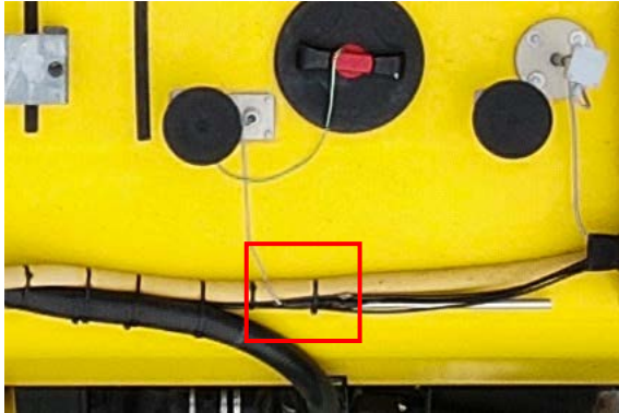
Abb. 128. DTP-Verbindung Frischwasser-Füllstandssensor
