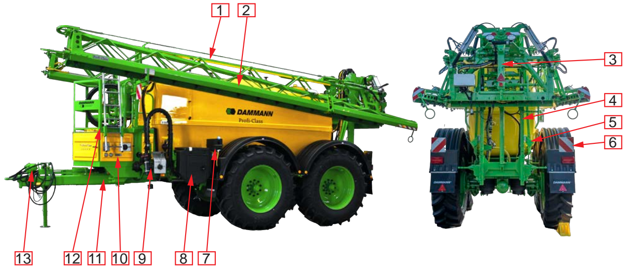
Abb. 3. Geräteübersicht
