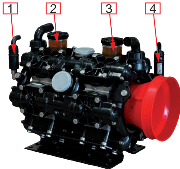
Abb. 33. Flüssigkeitspumpe AR 500
