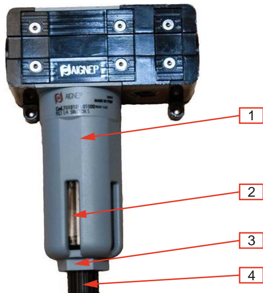
Abb. 127. Wartungseinheit
