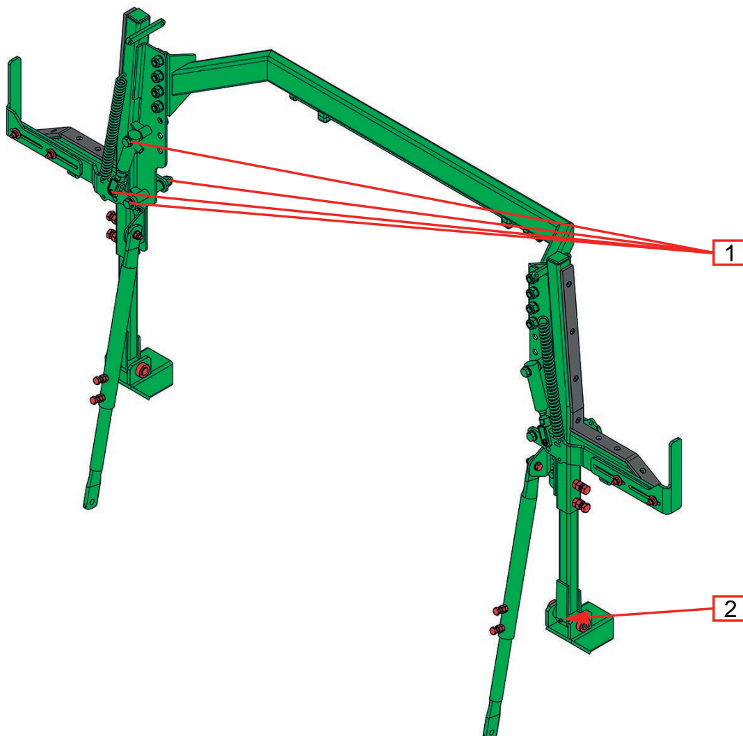
Abb. 122. Schmierplanübersicht Ablage
