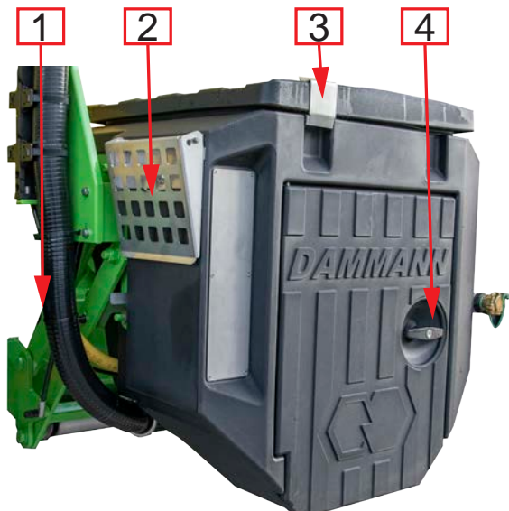
Abb. 30. Einspülzentrum 60 l
