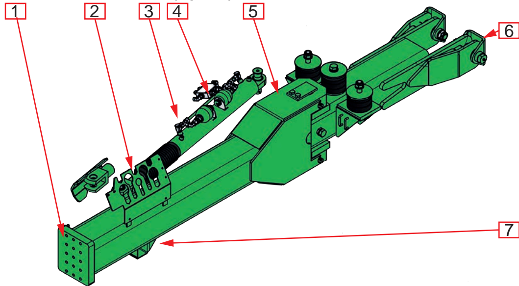
Abb. 7. Lenkdeichsel
