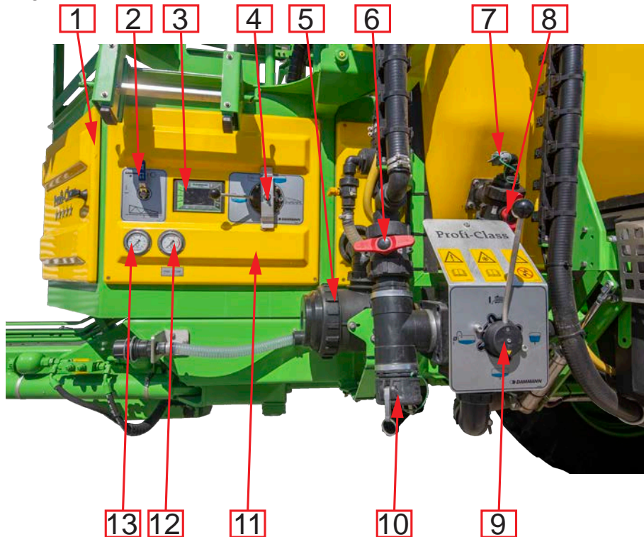
Abb. 27. Übersicht Armaturen und Hähne
