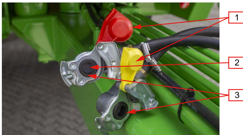
Abb. 41. Pneumatikkupplungen
