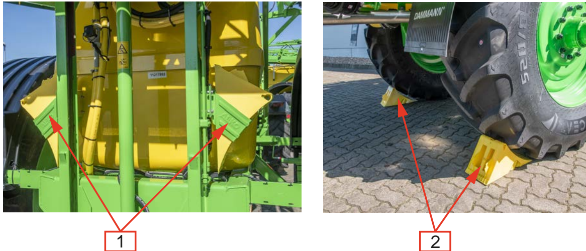
Abb. 59. Unterlegkeile
