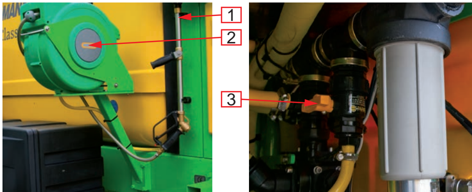
Abb. 36. Vario-Spritzrohr
