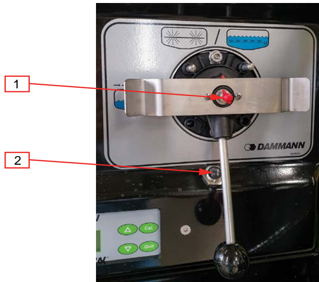
Abb. 118. Programmhahn Beispiel
