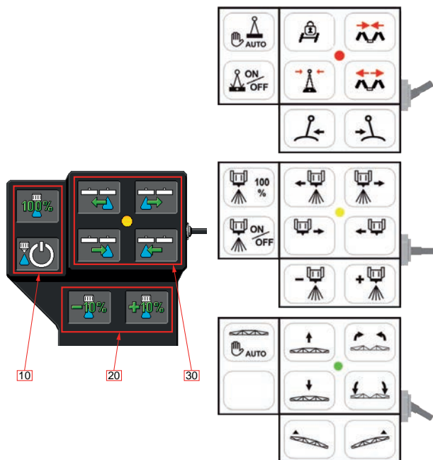
Abb. 46. Multifunktionsgriff
