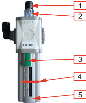
Abb. 125. Nebelöler
