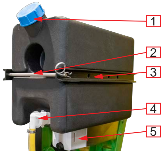
Abb. 32. Handwaschbehälter
