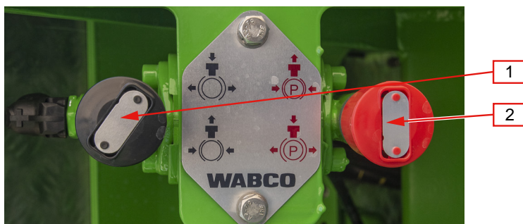
Abb. 39. Doppellöseventil
