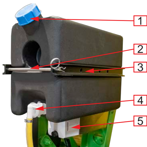
Abb. 64. Handwaschbehälter
