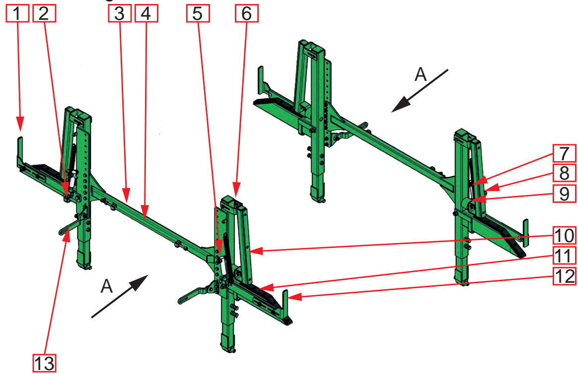
Abb. 5. Ablage
