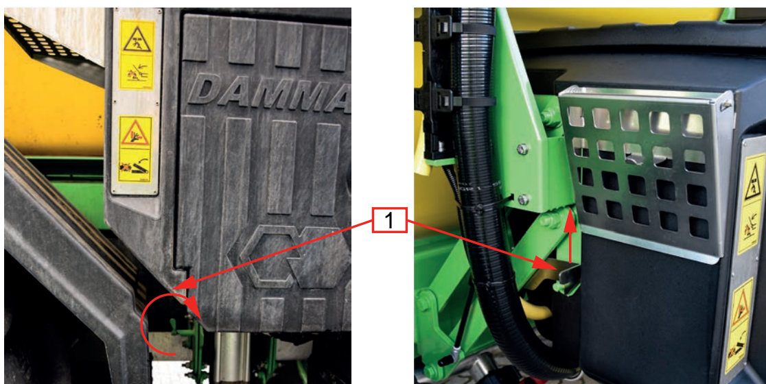
Abb. 62. Sicherung (pneumatisch links/mechanisch rechts)
