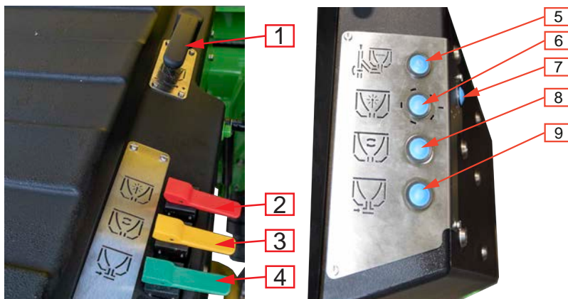
Abb. 63. Einspülzentrum 60 Liter (Tastenbelegung je nach Ausführung)
