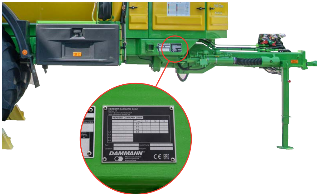
Abb. 2. Fahrzeug-Identifikation
