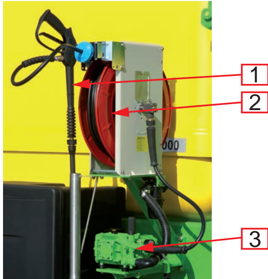
Abb. 38. Hochdruckreiniger Profi-Class
