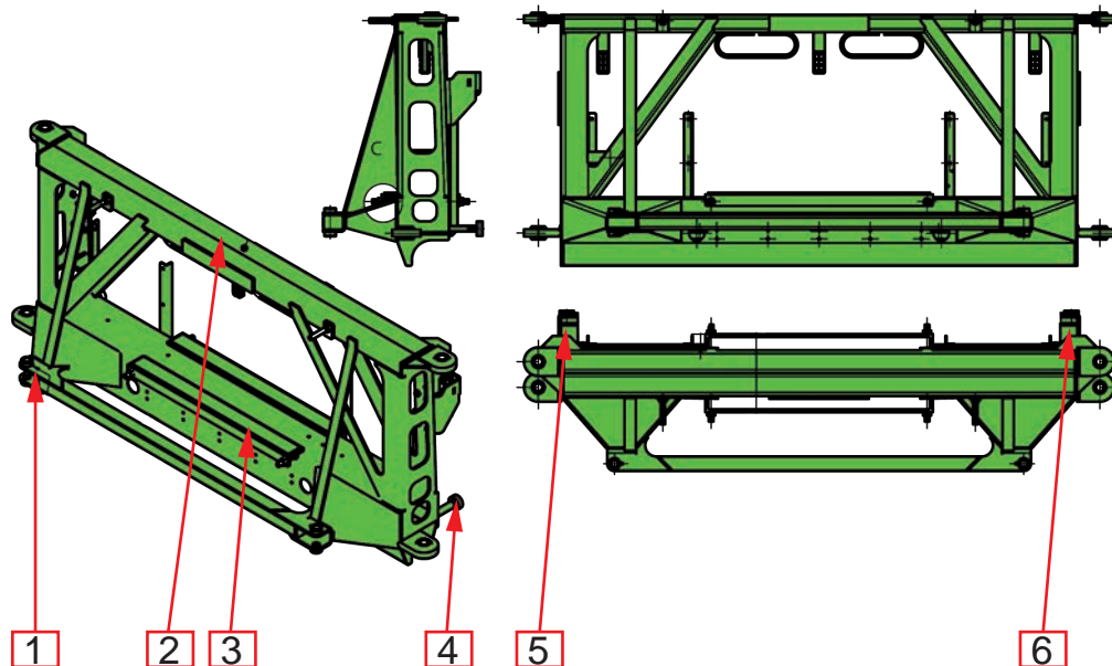
Abb. 14. Mittelrahmen
