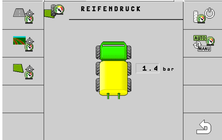
Abb. 68. Funktion der Reifendruckregelanlage
