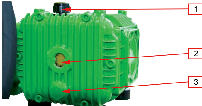
Abb. 109. Ölablassschraube/Öleinfüllstutzen/Ölschauglas Hochdruckreiniger
