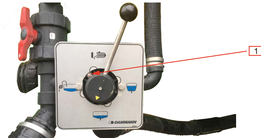
Abb. 117. Saughahn ANP
