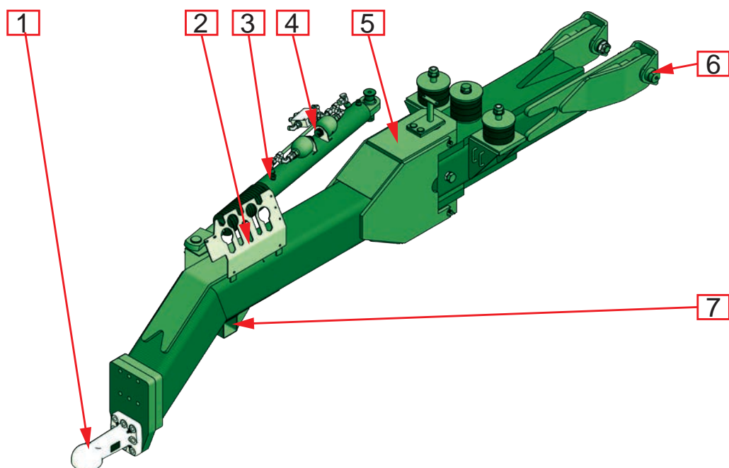
Abb. 8. Untere Lenkdeichsel
