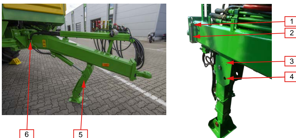
Abb. 51. Hydraulischer Stützfuß, links Untenanhängung, rechts Obenanhängung
