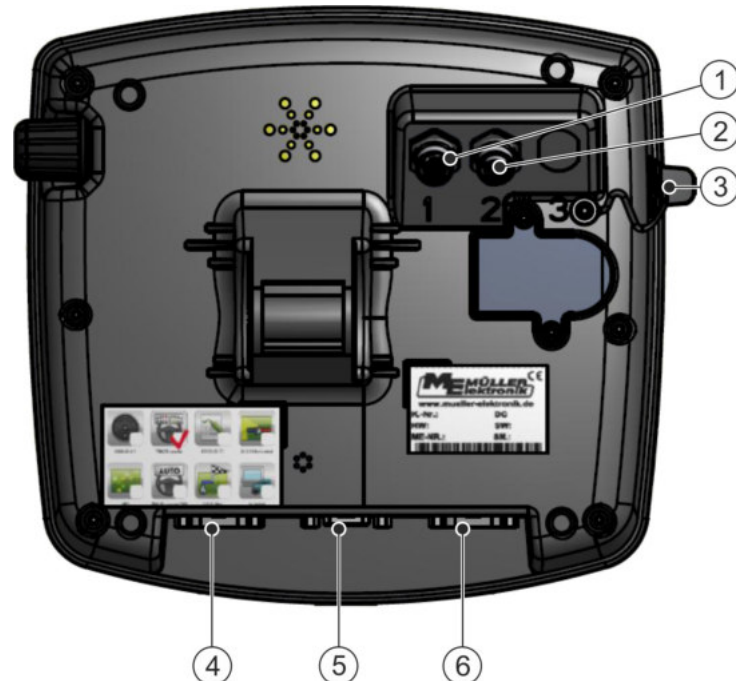
Zadní strana terminálu. Variant s připojením k kamery
