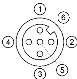
Obsazení kolíků zdiřky (v terminálu)
