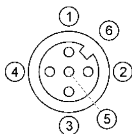
Pinbezetting van de bussen (in de terminal)
