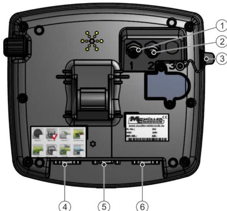
Achterkant van de terminal. Variant met en camera-aansluitingen
