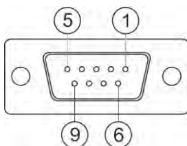
9-полюсна Sub-D бужса
