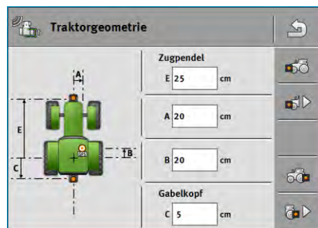
Beispielhafte Traktorgeometrie
