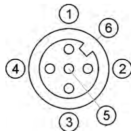
M12-Buchse: Kamera
