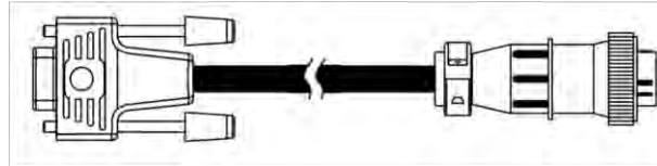
Anschlusskabel D-Sub <-> CPC Art.-Nr. 30322541
