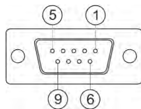
9 polių „Sub-D“ kištukinis lizdas
