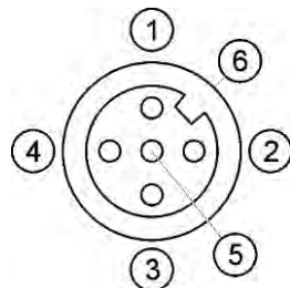
M12 kištukinis liždas: Kamera
