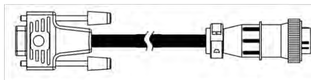
Připojovací kabel D-Sub <-> CPC číslo artiklu 30322541
