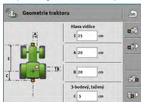
Příkladná geometrie traktoru
