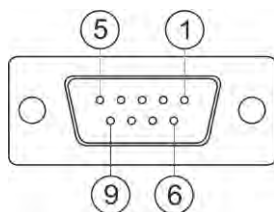
9-pólová zdiřka D-Sub
