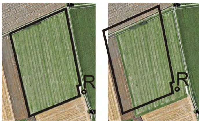
Stânga - câmp cu o poziție GPS calibrată; dreapta - câmp fără o poziție GPS calibrată
